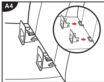
③ 将两个ISOFIT安装导向件对准刚性固定点后插入。
